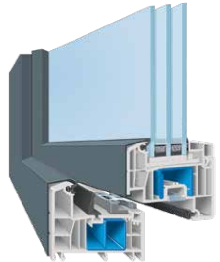
AFINO-top MD (Mitteldichtungssystem mit drei Dichtungen)
