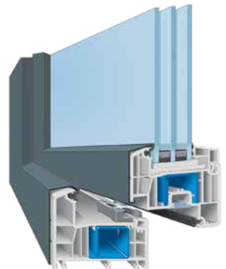
AFINO-top AD (Anschlagdichtungssystem mit zwei Dichtungen)
