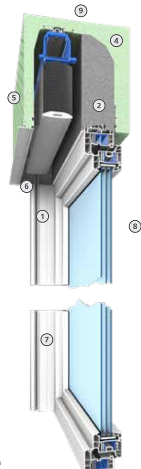
Eingeschäumte Stabilisatoren
